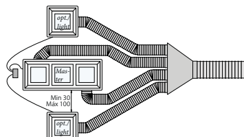
Installation: exempel med 2 moduler
