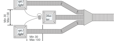
Installation: eksempel med 3 moduler
