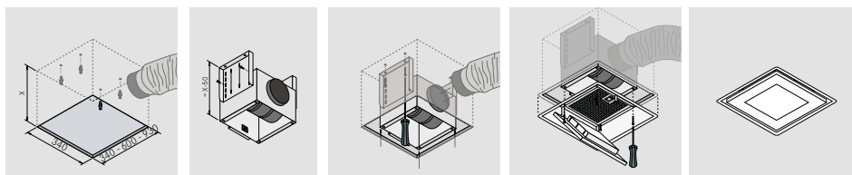
Enkel installation vid montering på plattan från utskärningen på det nedsänkta taket
